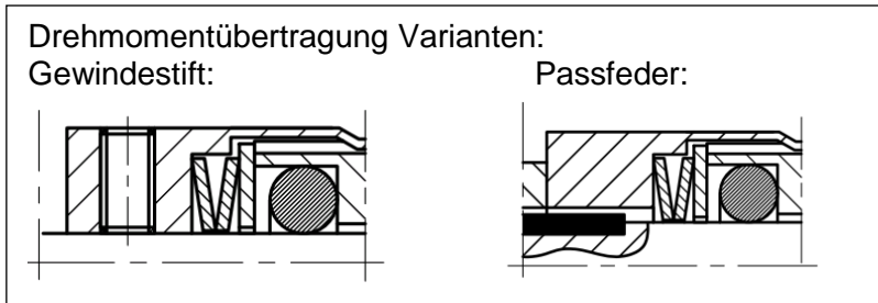
Beispielszeichnung mit Gegenring ASP-952-G
