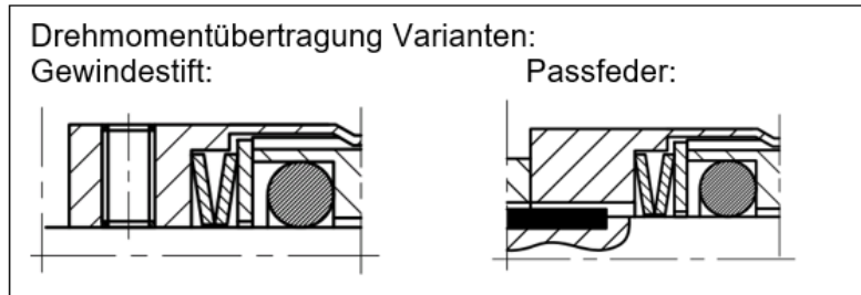
Beispielszeichnung mit Gegenring ASP-952-G
